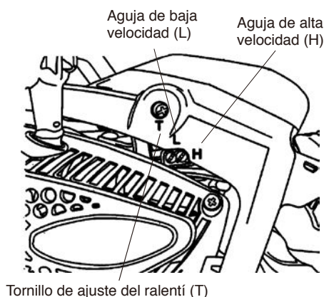
Tornillo de ajuste del ralentí (T)
